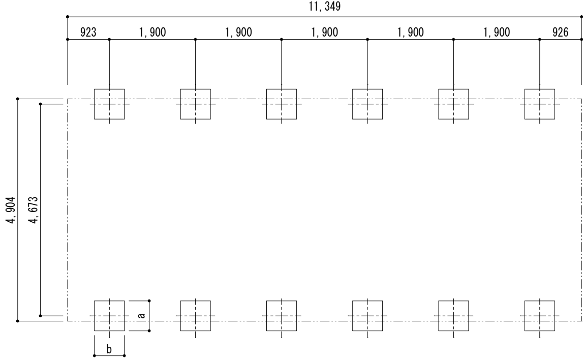
■基礎配置図
